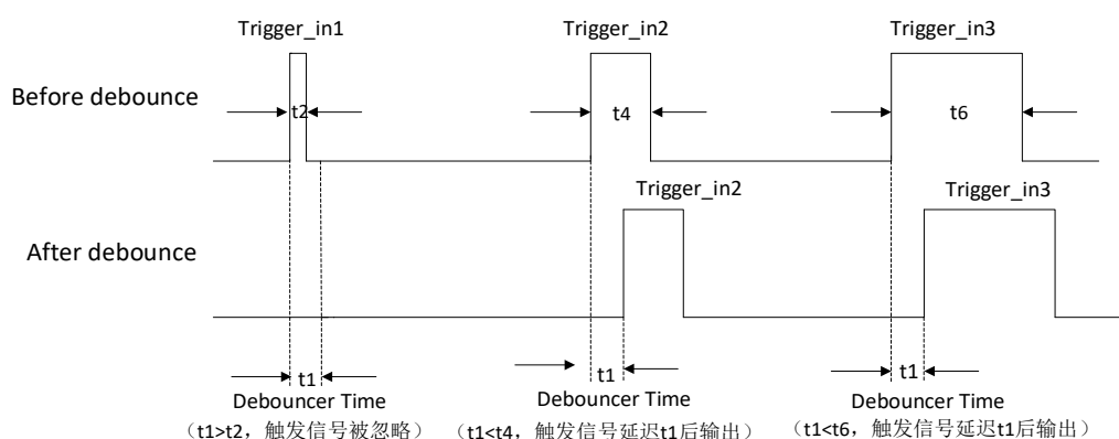
图3-16 触发输入信号去抖时序
