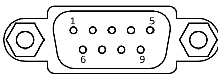
图4-26 9-pin 公头连接器
