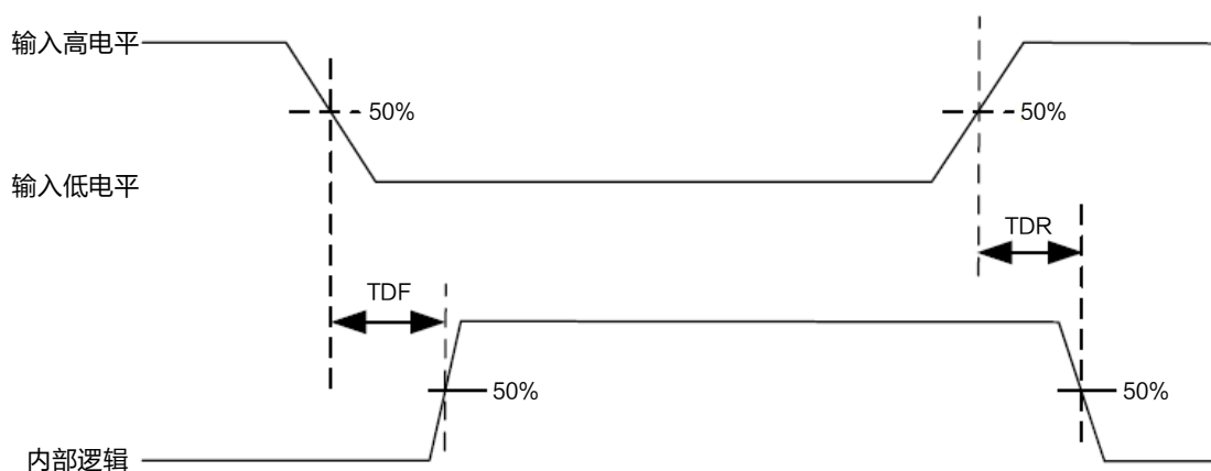
图4-12 输入逻辑电平
