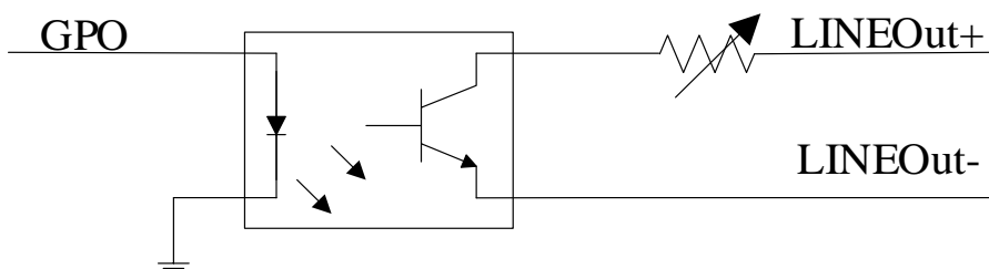
图4-14 输出内部电路图
