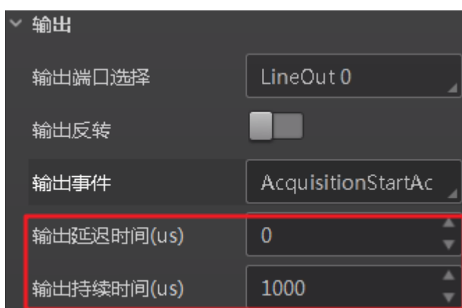
图3-26 光耦输出设置
