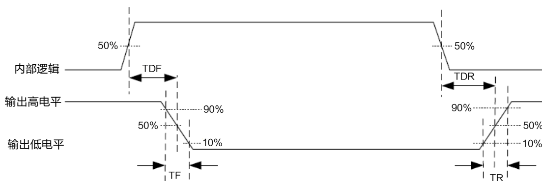
图4-15 输出逻辑电平
