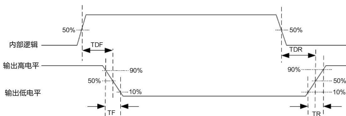
图4-4 输出逻辑电平
